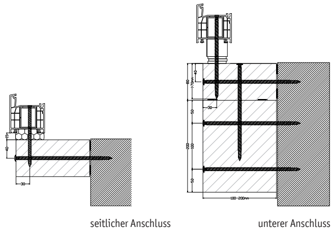
seitlicher Anschluss unterer Anschluss
