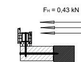
seitlicher Anschluss, weite Ausladung
