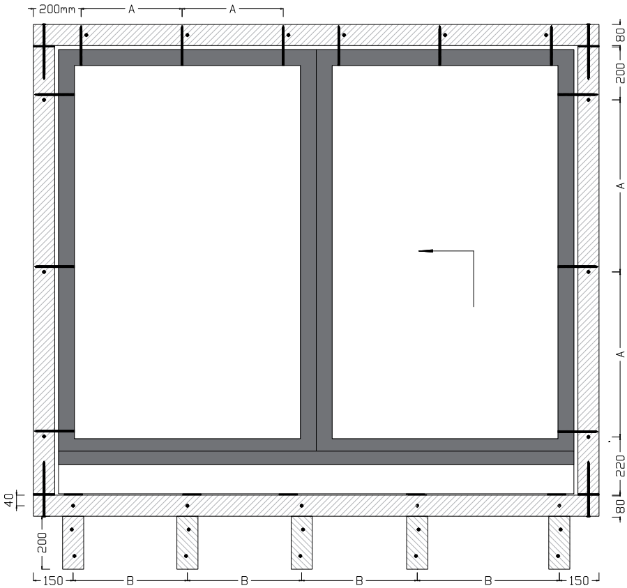
unterer Anschluss unterer Anschluss Verschraubung von unten: Verschraubung von oben:
