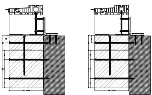
unterer Anschluss unterer Anschluss Verschraubung von unten: Verschraubung von oben:
